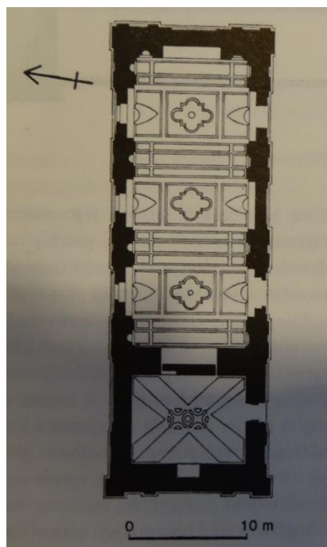
Il. 5. Kościół św. Agnieszki, rzut poziomy, plan 1:500, Źródło: A. Miłobędzki, Architektura polska XVII wieku . Warszawa 1980, s. 245.
